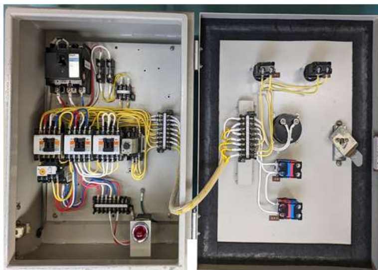
盤内図(補助接点ユニットあり)
