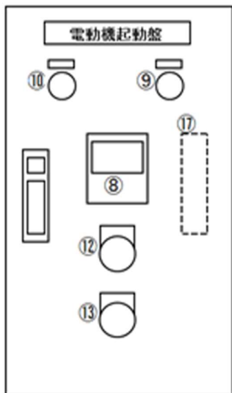
盤面 正面図
