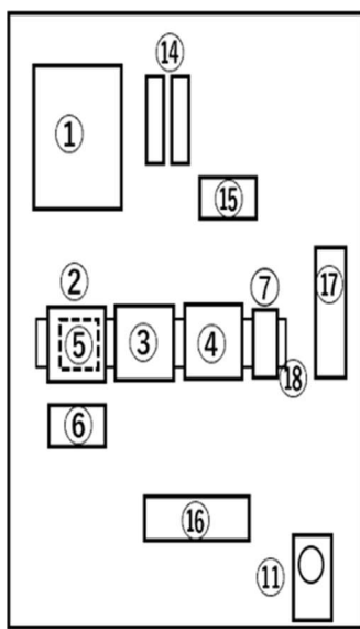
盤内部品配置図
