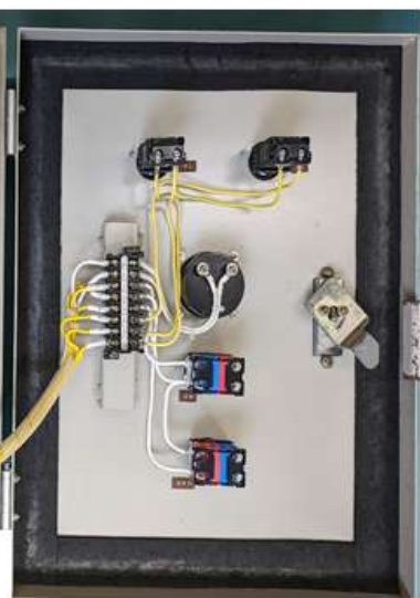
盤裏面
